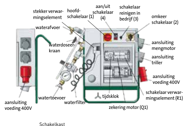
Schakelkast
