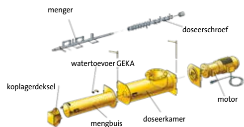
Doorstroommenger
