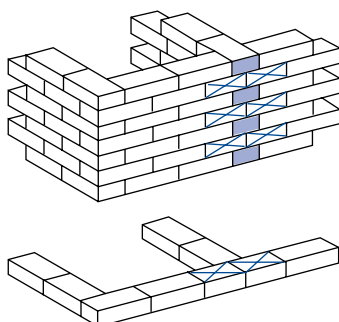
[Fig 12] Hoekoplossing in ontmoeting met halfsteensverband
