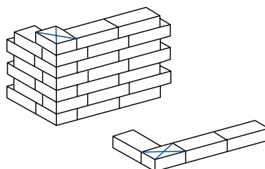
[Fig 13.1] Hoek in staand klezorenverband uitgevoerd
