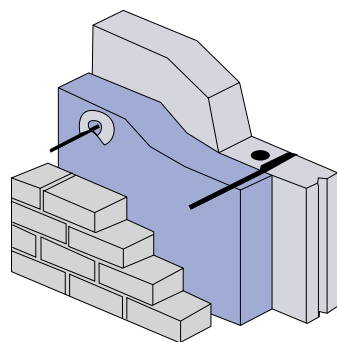
[Fig 16] Spouwmuur met binnenblad van kalkzandsteenlijmwerk.
