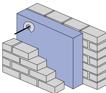
[Fig 17] Spouwmuur met gemetseld binnenblad.
