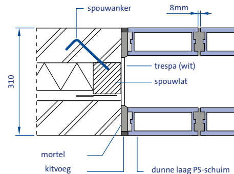
[Fig 24] Aansluiting van glazen bouwsteen aan metselwerk
