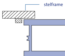
[Fig 23] Houten stelframe
