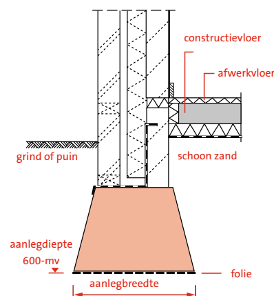
[Fig 3] Fundering van stampbeton gemaakt met schuif- of glijbekisting.
