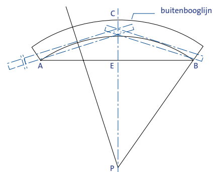
[Fig 30] Trekken van een segmentboog.
