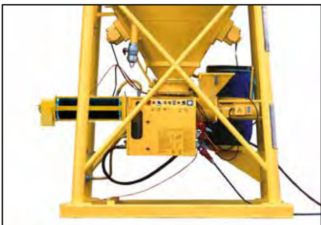
Doorstroommenger SM D100ru en D150ru
