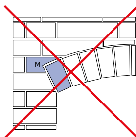
[Fig 29.2] Zijaansluiting (aanzet) van segmentboog
