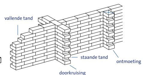
[Fig 13.2] Muurfragment met ontmoeting, doorkruising en beëindigingen in staand klezorenverband
