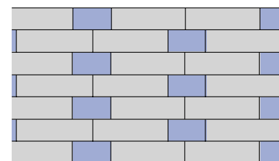
[Fig 11] Kettingverband in halfsteenswerk
