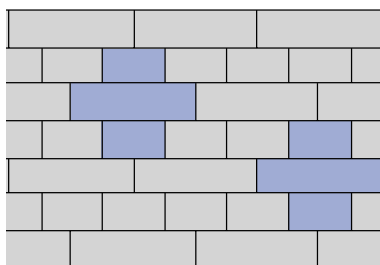
[Fig 9] Kruisverband in aanzicht
