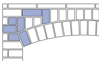
[Fig 29.5] Segmentboog zonder lange scherpe punten in het aansluitende metselwerk
