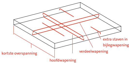
[Fig 5] Plaatbewapening in schema.
