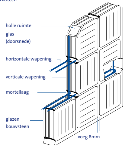
[Fig 22] RVS betonstaal in de voegen van glazen bouwstenen
