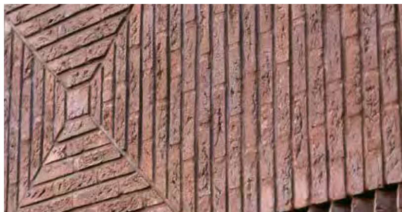
[Fig 14] Waterkerende laag met open stootvoegen
