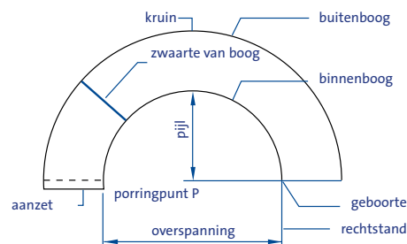
[Fig 26] Halfrondboog met benamingen
