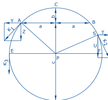
[Fig 27] Segmentboog en ontbinding van krachten bij rond- en segmentbogen
