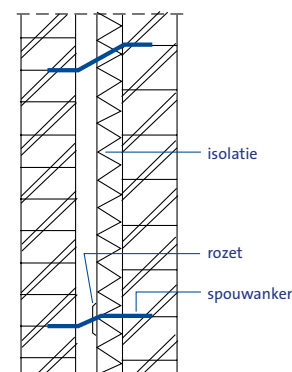
[Fig 15] Spouwankers altijd afwaterend aangebracht, ook bij ongelijke laagverdeling
