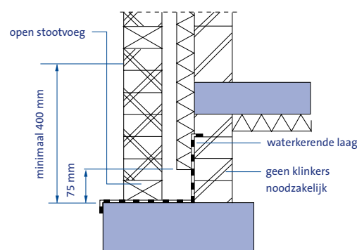
[Fig 14] Waterkerende laag met open stootvoegen
